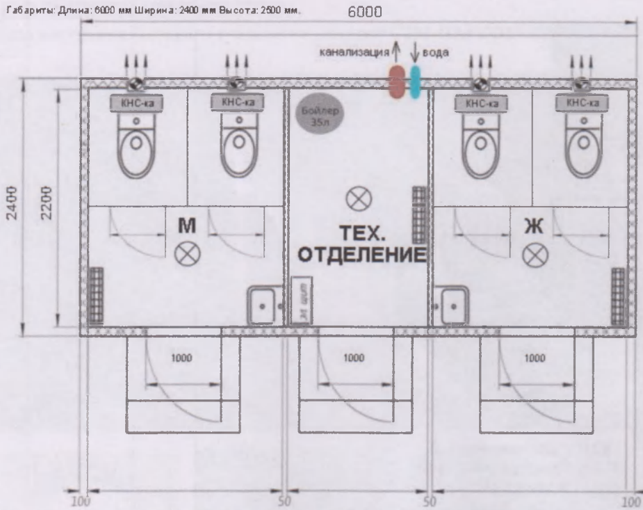
Комплектующие сетевого туалетного модуля "СТМ-ПАРКОВЫЙ-2МЖ1Т"
